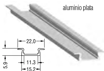
PERFIL Aluminium EMPOTRADO PARA LEDS 2000 x 22 nº1 Cod. L02001000
