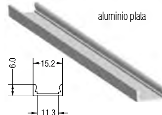
PERFIL Aluminium DE SUPERFICIE PARA LEDS 2000 x 15 nº2 Cod. L02002000
